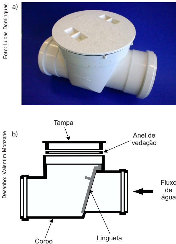
Figura 7. a) Válvula de retenção de PVC, b) Desenho esquemático da válvula de retenção.
